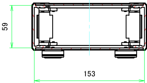
B-B ( 1:3 )
