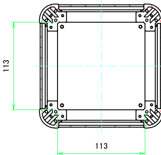
C-C ( 1:3 )
